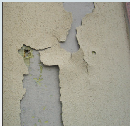
Отслоение декоративного покрытия вследствие воздействия большого количества воды
