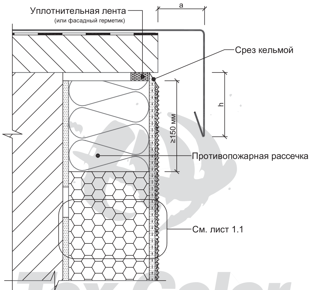
Рекомендуемые значения геометрических размеров козырька
