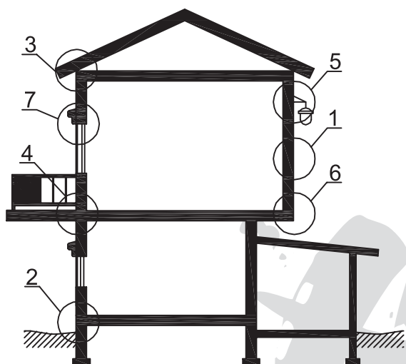
Схематический разрез типового дома (разделы 1-7)
